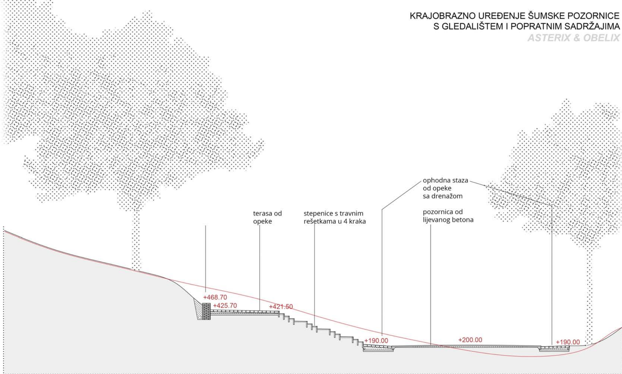
PRESJEK B
